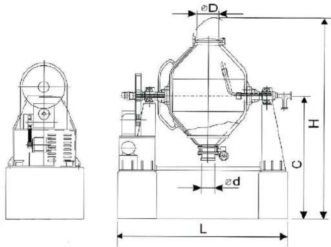
構造圖 (STRUCTURE DIAGRAM)
